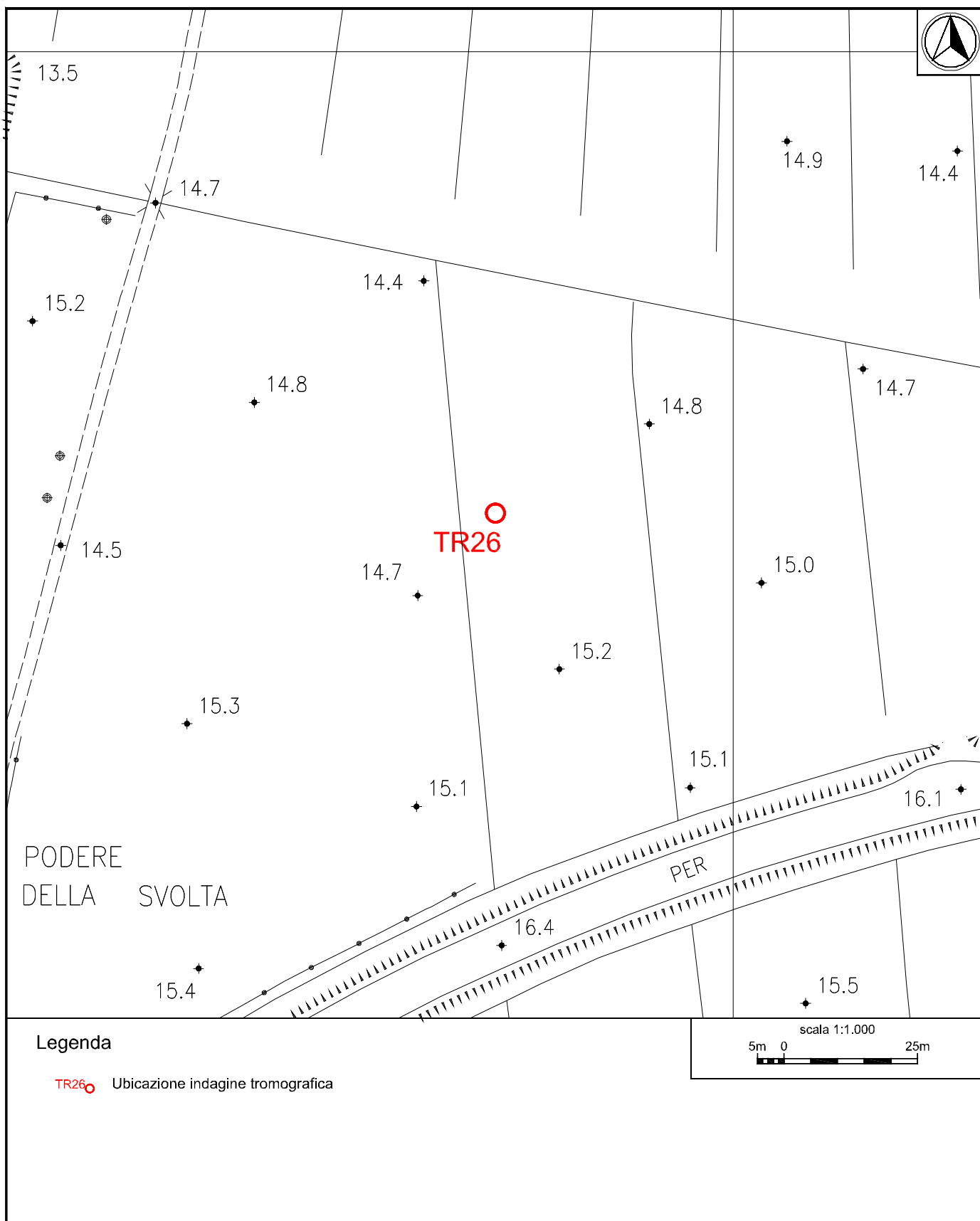
Ubicazione indagine in sismica passiva Sito 26. Dettaglio.
