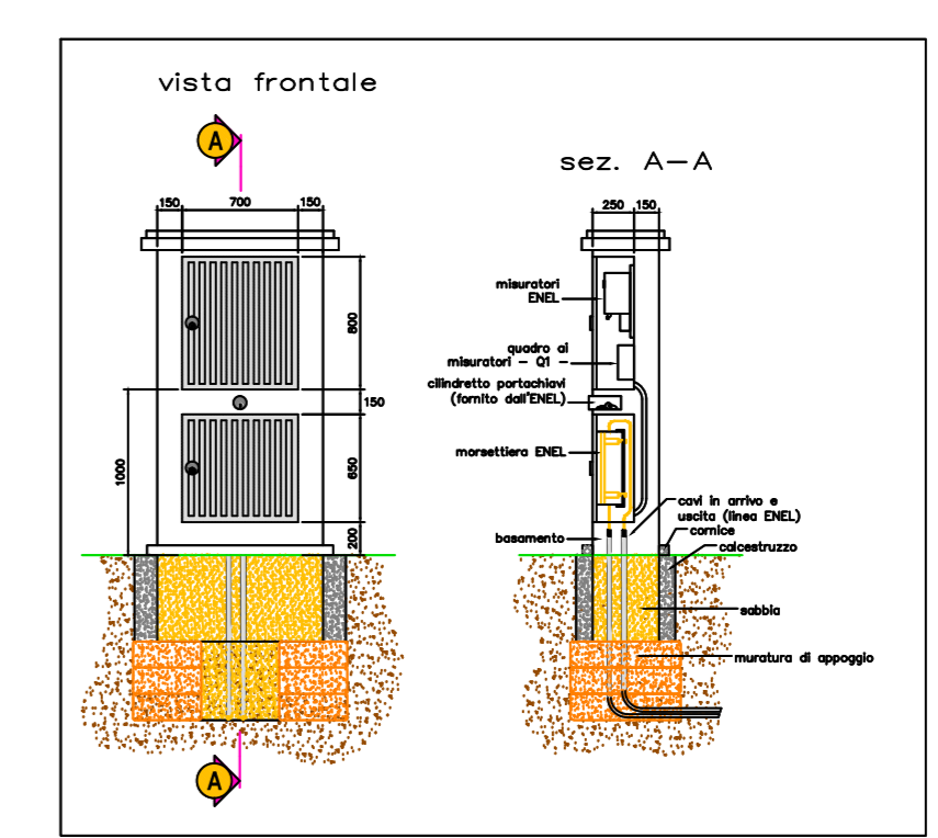
PARTICOLARE FORNITURA ENEL
