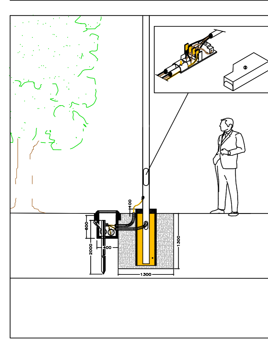
PARTICOLARE BASE PALO
