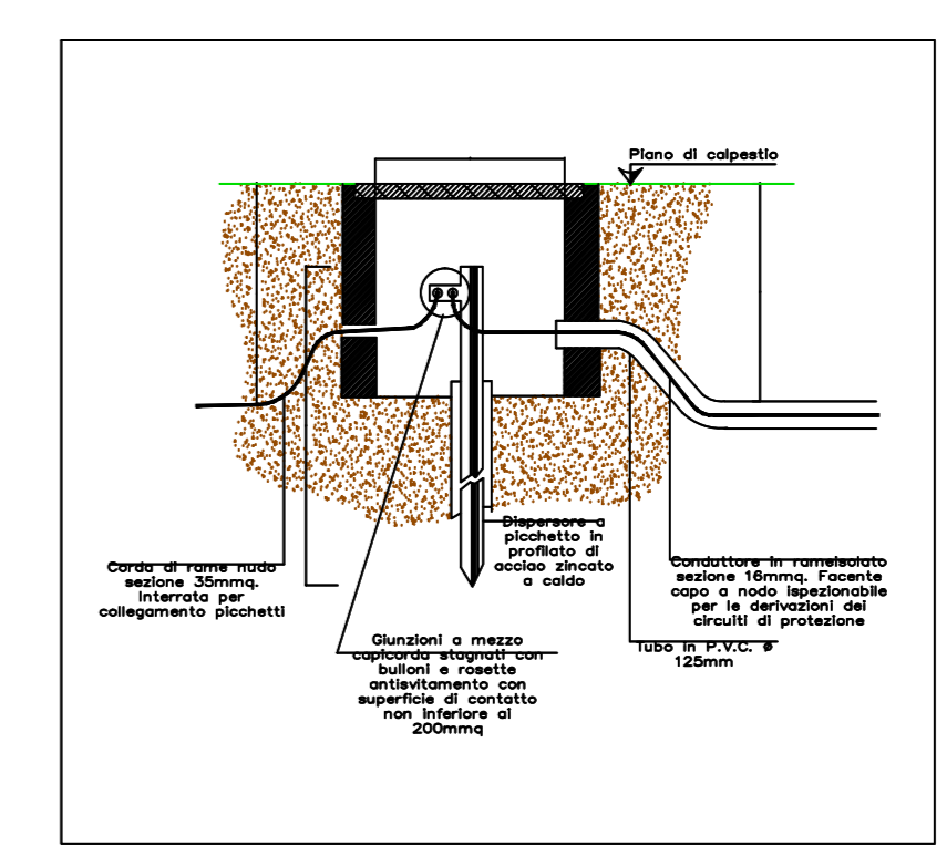
PARTICOLARE DISPENSORE DI TERRA
